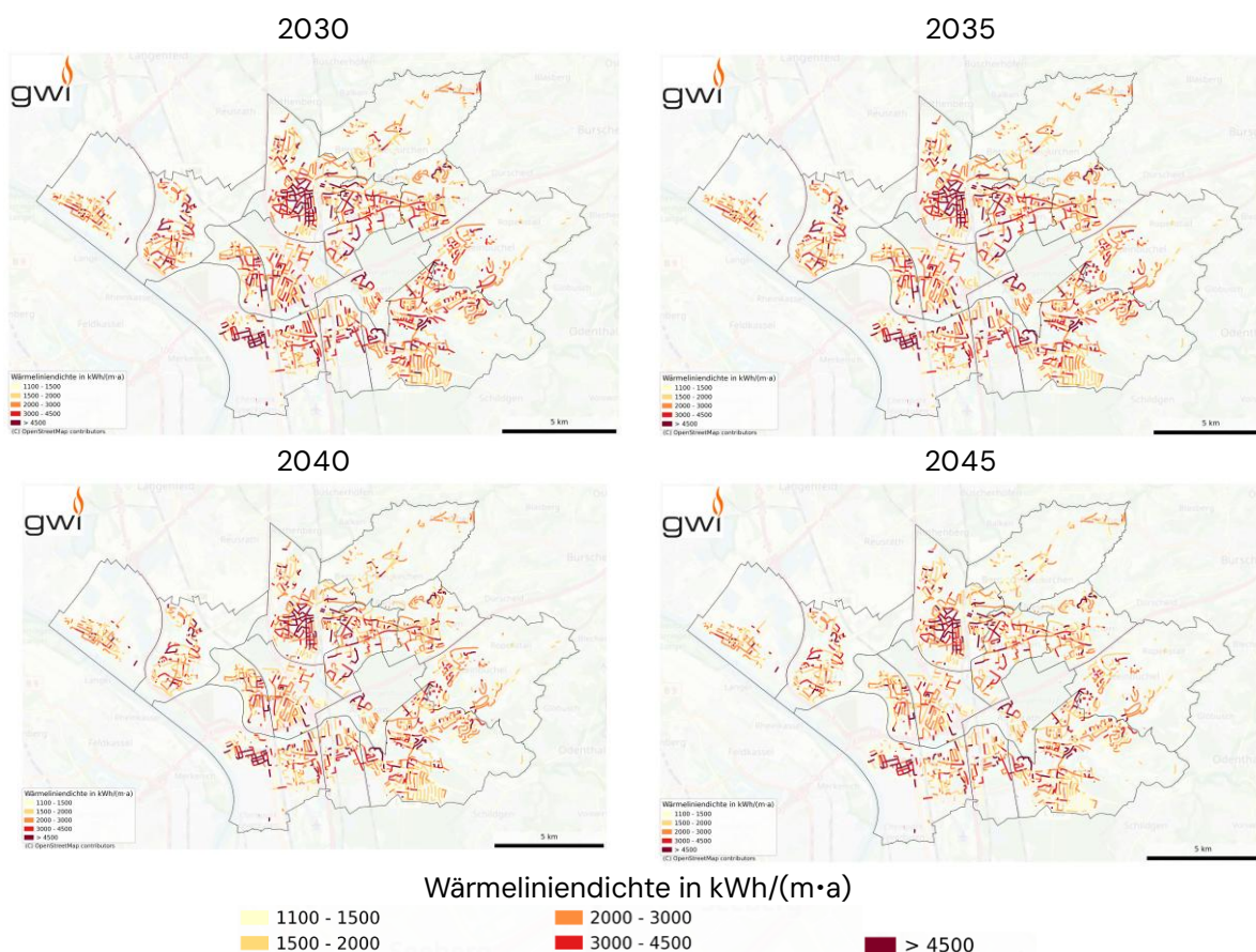
Abbildung 76: Wärmelinienendichten im maßgeblichen Zielszenario. Gebiete mit ausschließlich industrieller Nutzung wurden nicht berücksichtigt (Quelle: ALKIS , LANUK-BB )
