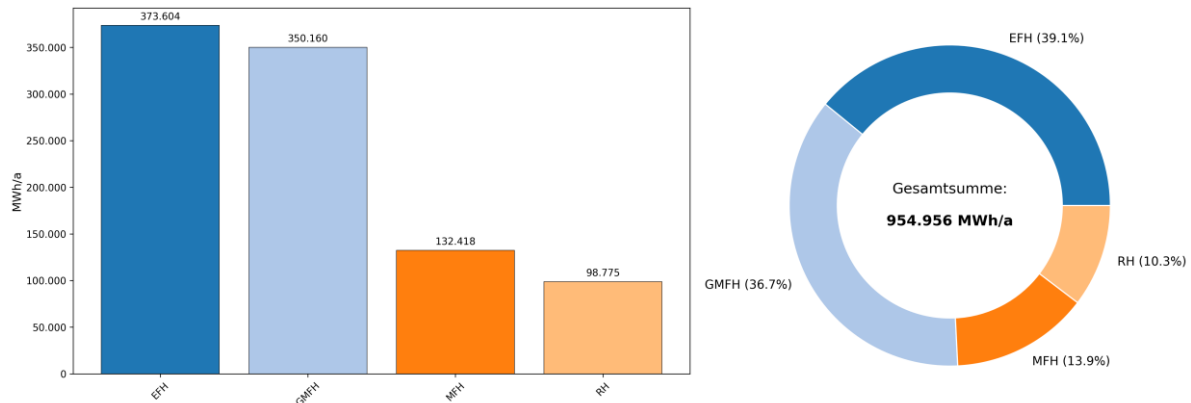
Abbildung 22: Verteilung des Nutzenergiebedarfs nach Wohngebäudeart (Quellen: ALKIS , LANUK-RBM , RNG-RLM , RNG-EFH/MFH , RNG-NSH/WP , EVL-FW )
