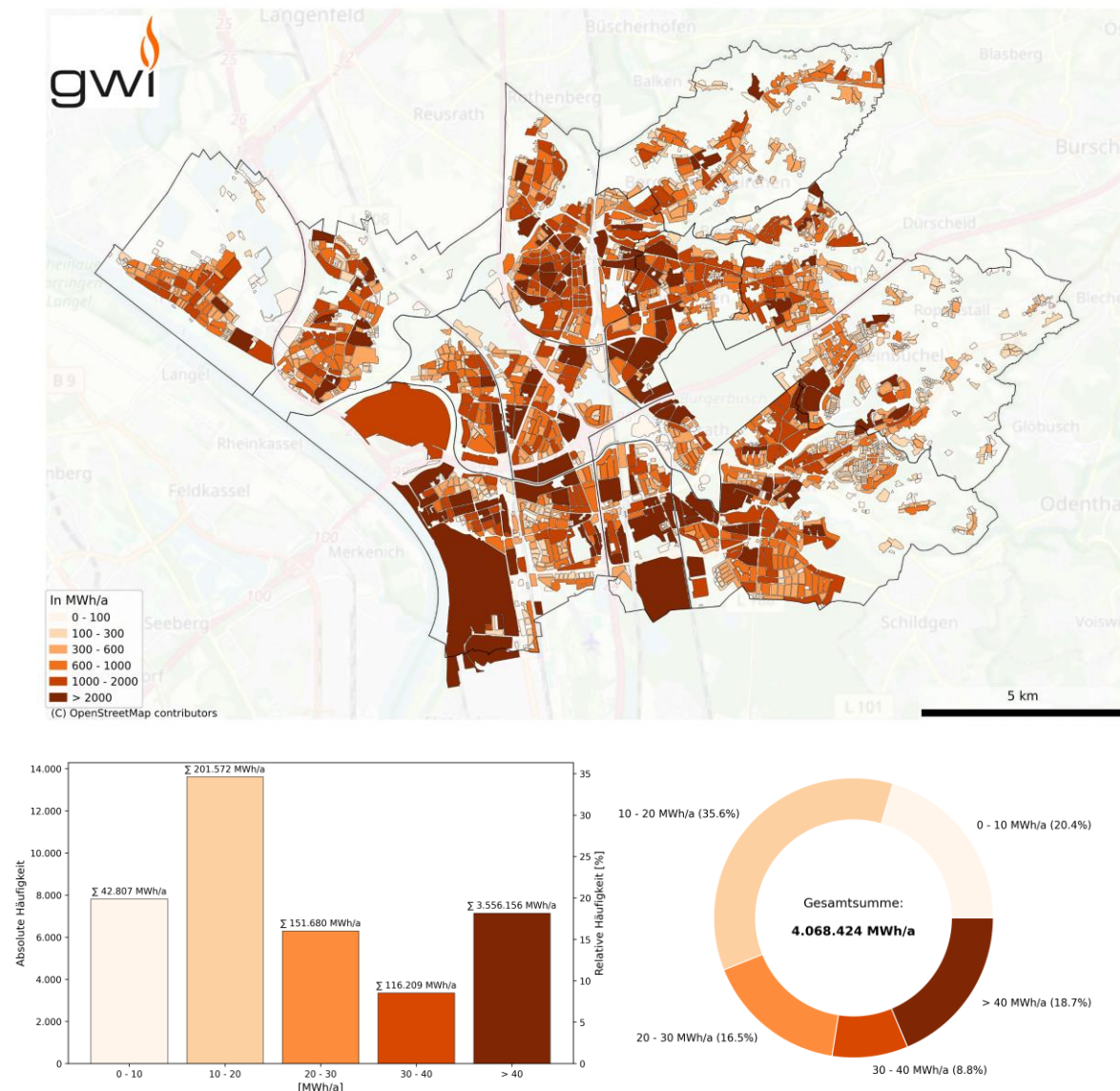
Abbildung 38: Endenergiebedarfe im Baublock sowie deren statistische Verteilung auf Gebäudeebene (Quellen: ALKIS , LANUK-BB , RNG-RLM , RNG-EFH/MFH , RNG-NSH/WP , EVL-FW , CHEM , KD , TK )
