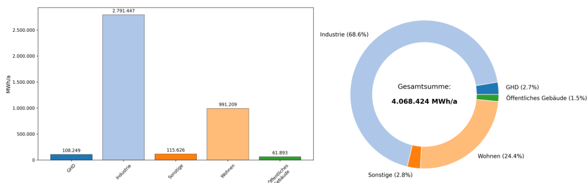
Abbildung 41: Verteilung des Endenergiebedarfs auf die einzelnen Sektoren (Quellen: ALKIS , LANUK-RBM , RNG-RLM , RNG-EFH/MFH , RNG-NSH/WP , EVL-FW , CHEM , KD , TK )
