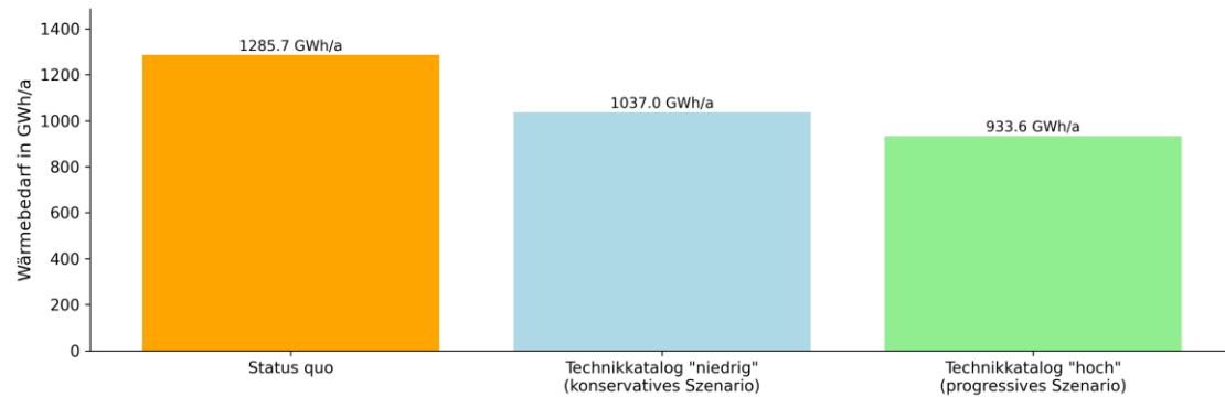
Abbildung 52: Wärmebedarfsentwicklung: Status quo und theoretische Reduktionspotenziale durch Gebäudesanierung (Quellen: RNG-RLM , RNG-EFH/MFH , RNG-NSH/WP , EVL-FW , TK )
