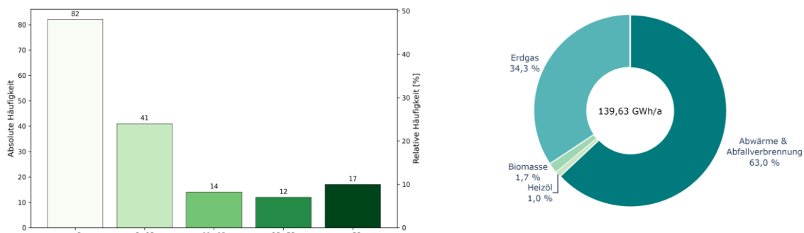
Abbildung 37: Wärmenetzversorgte Baublöcke und Wärmenetz (rot), sowie statistische Verteilung der Baublöcke im Balkendiagramm und Speisung der Wärmenetze im Donutdiagramm (Quellen: ALKIS , LANUK-BB , EVL-FW )
