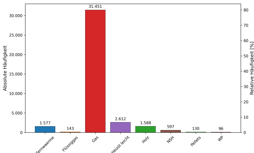
Abbildung 26: Technologieverteilung der beheizten Gebäude (Quellen: ALKIS , KD , RNG-EFH/MFH , RNG-RLM , RNG-NSH/WP , EVL-FW )
