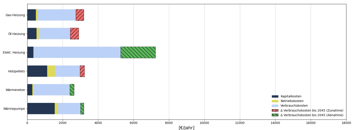
Abbildung 89: Mehrfamilienhaus saniert. Wohnfläche = 300m², Wärmeleistung = 8,8 kW, Wärmebedarf = 15 MWh/a (eigene Darstellung)
