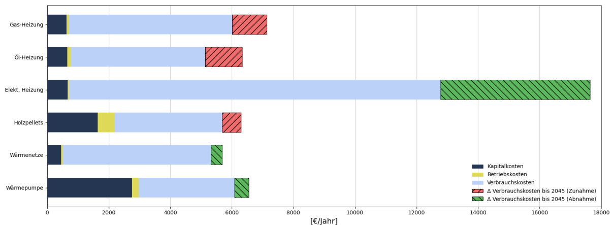
Abbildung 88: Mehrfamilienhaus unsaniert. Wohnfläche = 300m², Wärmeleistung = 20,5 kW, Wärmebedarf = 37 MWh/a (eigene Darstellung)
