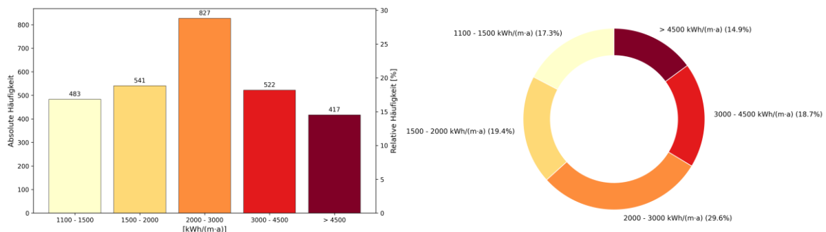
Abbildung 25: Wärmelinien und statistische Verteilung der Straßenabschnitte (Quellen: ALKIS , LA-NUK-RBM , RNG-RLM , RNG-EFH/MFH , RNG-NSH/WP , EVL-FW )
