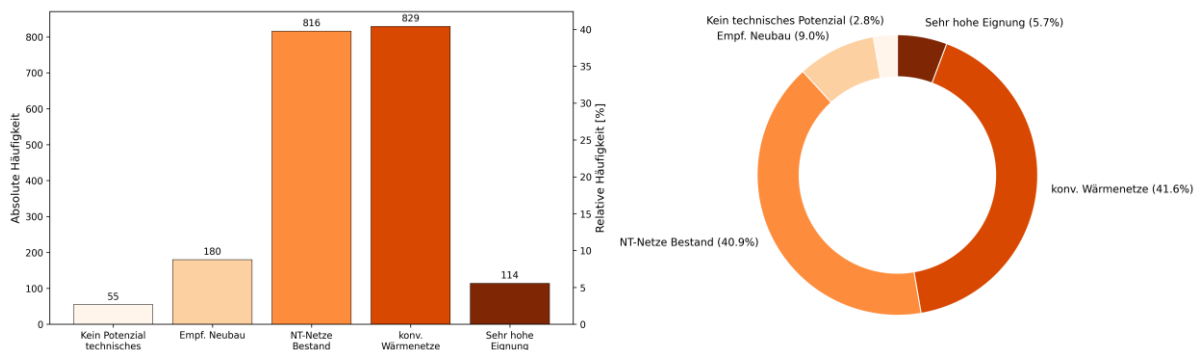
Abbildung 47: Eignungsklassifikation der Baublöcke nach KEA-BW inkl. Bestandsnetze (grün) sowie statistische Verteilung der Baublöcke (Quellen: ALKIS , LANUK-BB , LANUK-RBM , RNG-RLM , RNG-EFH/MFH , RNG-NSH/WP , EVL-FW )
