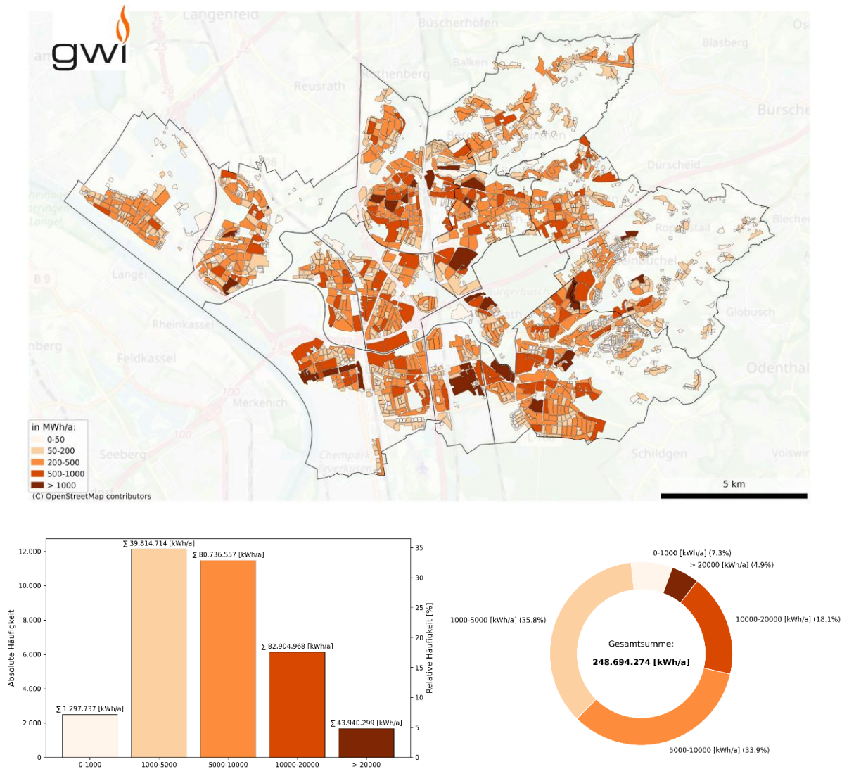
Abbildung 51: Potenzielle Raumwärmebedarfsreduktion durch Sanierungsmaßnahmen nach Szenario „Technikkatalog niedrig“ (Quellen: ALKIS , LANUK-BB , RNG-RLM , RNG-EFH/MFH , RNG-NSH/WP , EVL-FW , TK )
