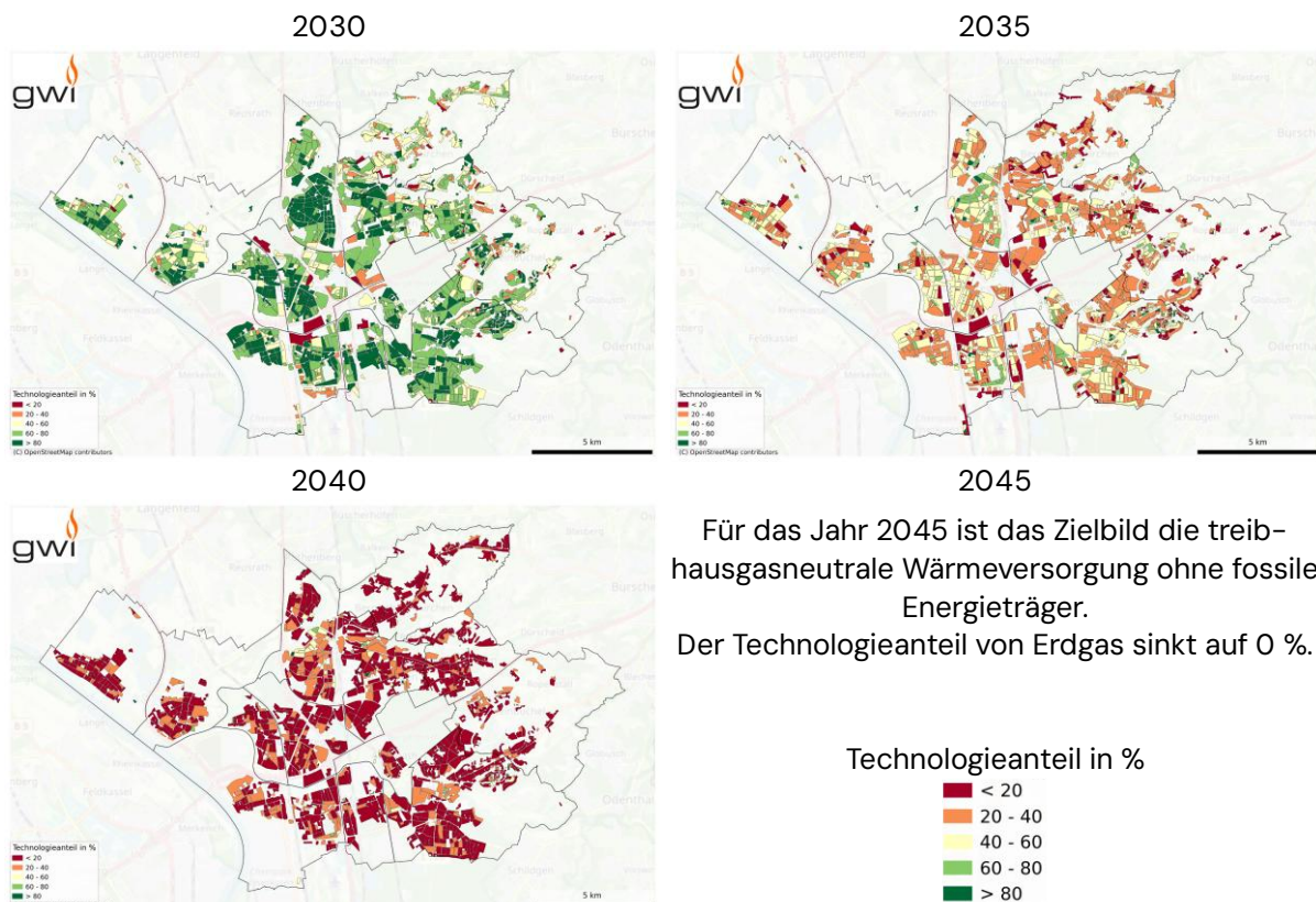
Abbildung 67: Erdgasversorgung im maßgeblichen Zielszenario als Technologieanteil Erdgas. Baublöcke mit ausschließlich industrieller Nutzung wurden nicht berücksichtigt (Quelle: ALKIS , LANUK-BB )
