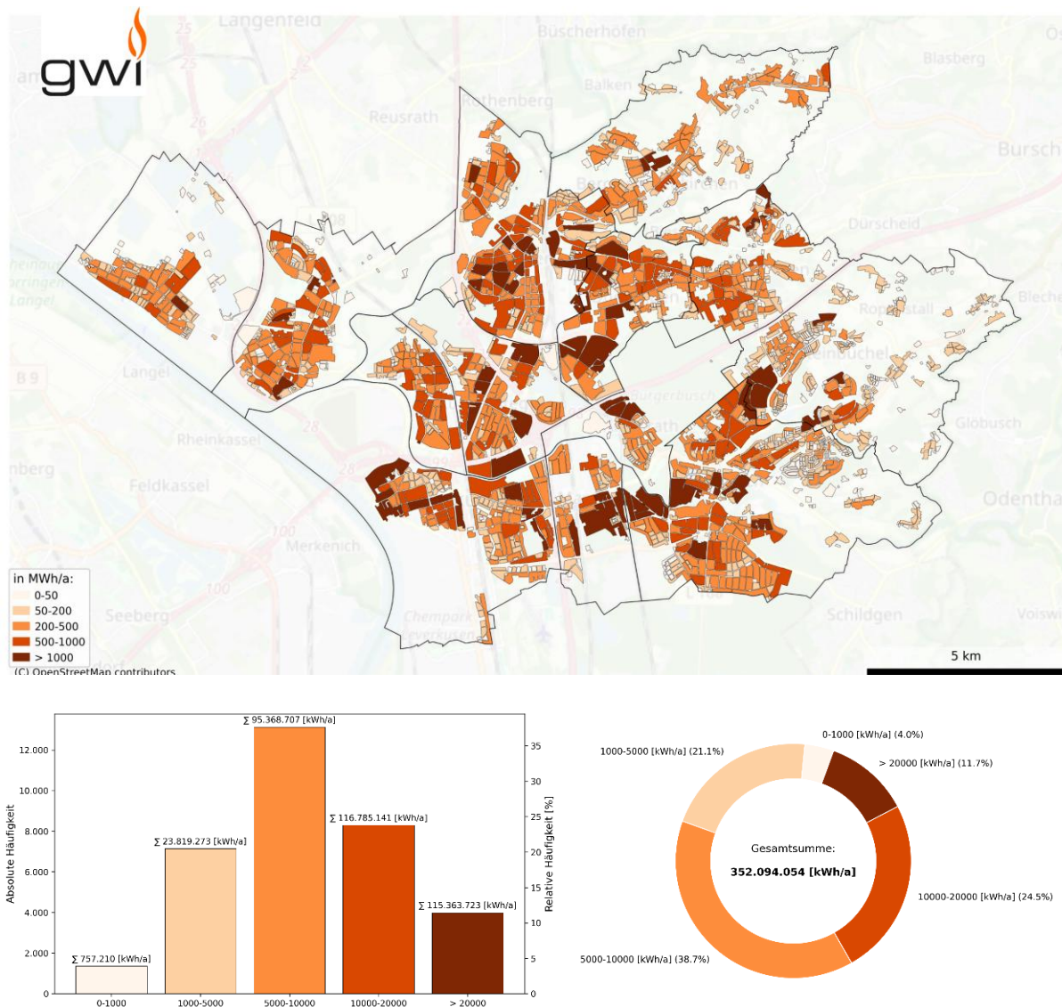
Abbildung 50: Potenzielle Raumwärmebedarfsreduktion durch Sanierungsmaßnahmen nach Szenario „Technikkatalog hoch“ (Quellen: ALKIS , LANUK-BB , RNG-RLM , RNG-EFH/MFH , RNG-NSH/WP , EVL-FW , TK )
