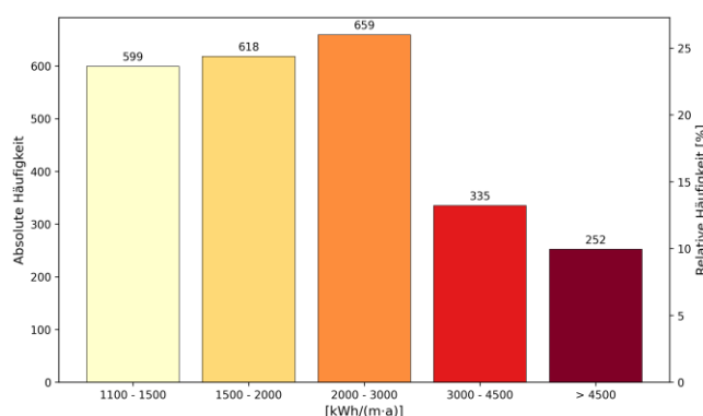
Abbildung 77: Häufigkeit der Wärmelinienendichten im maßgeblichen Zielszenario (2045) (eigene Darstellung)
