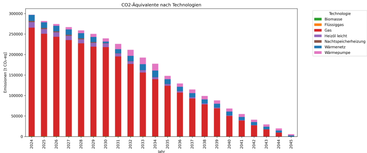
Abbildung 82: Jährliche Entwicklung der Treibhausgasemissionen der Gebäude nach Technologien im maßgeblichen Zielszenario (eigene Darstellung)
