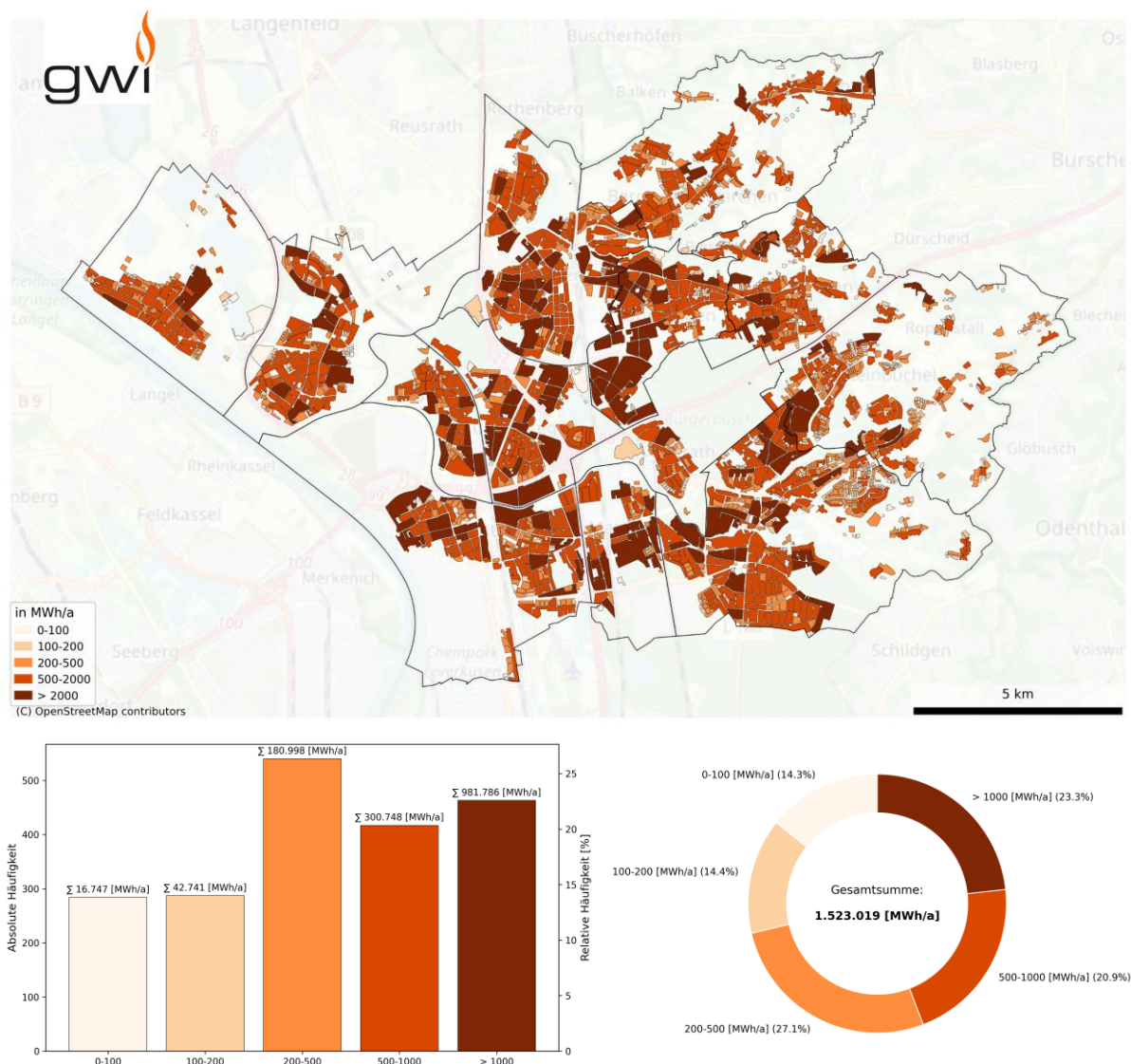
Abbildung 53: Dachflächen-Solarthermie Potenziale dargestellt auf Baublock-Ebene in MWh/a (Quellen: ALKIS , LANUK-BB , LANUK-DFST )
