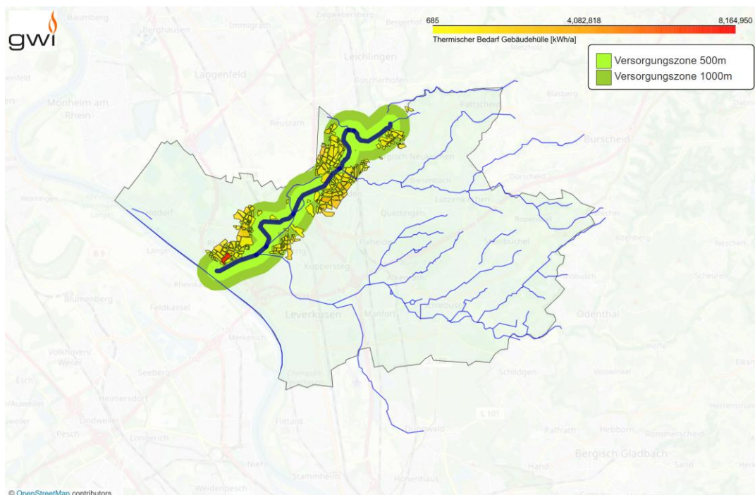
Abbildung 60: Teilausschnitt der Wupper mit Versorgungszonen (500 m Radius, 1000 m Radius) sowie Darstellung der Wärmebedarfe der Baublöcke innerhalb der Versorgungszonen (Quellen: ALKIS , LANUK-BB , RNG-RLM , RNG-EFH/MFH , AKG )
