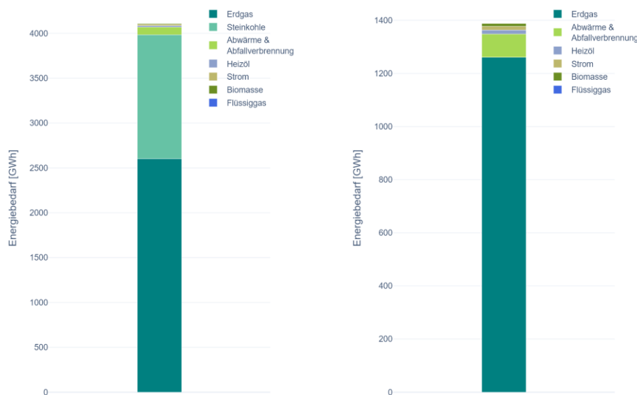
Abbildung 40: Eingesetzte Energieträger zur Wärmeerzeugung (Quellen: ALKIS , RNG-RLM , RNG-EFH/MFH , RNG-NSH/WP , EVL-FW , KD , CHEM , TK )
