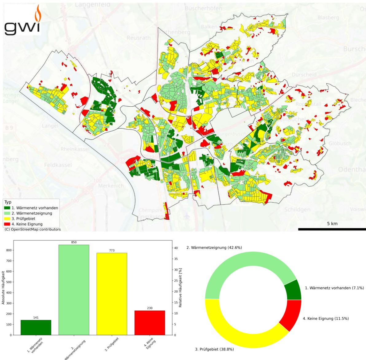
Abbildung 48: Erweiterte Eignungsklassifikation im Baublock sowie statistische Verteilung der Baublöcke (Quellen: ALKIS , LANUK-BB , LANUK-RBM , RNG-RLM , RNG-EFH/MFH , RNG-NSH/WP , EVL-FW )
