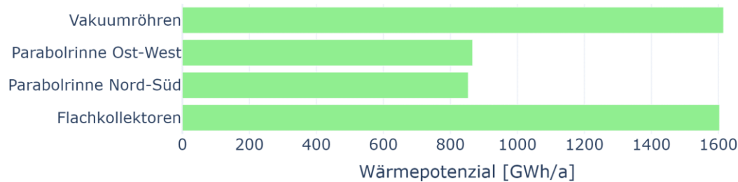
Abbildung 54: Potenzieller jährlicher Freiflächen-Solarthermie Wärmeertrag in GWh/a für unterschiedliche Technologieoptionen (Quelle: LANUK-DFST )
