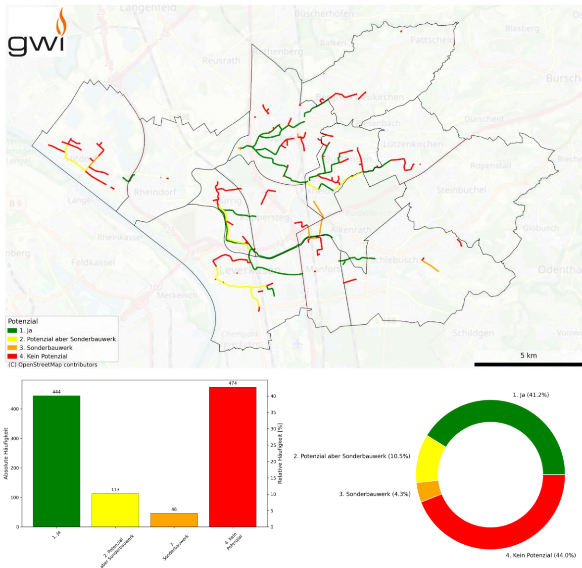
Abbildung 63: Kartografische Darstellung des Abwassersystems (Quelle: ABW )
